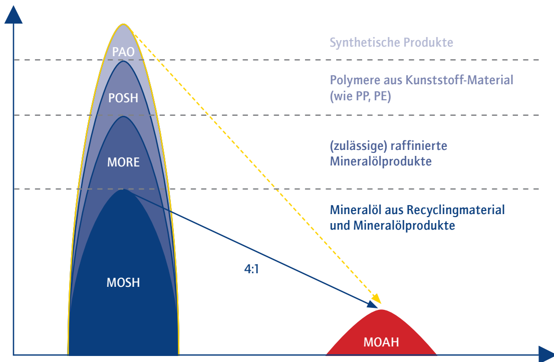
Abbildung 2: Verschiebung des im Mineralöl üblichen MOSH : MOAH-Verhältnisses durch MORE, POSH und PAO als MOSH-Analoga [nach 14 und 15] (Abkürzungen siehe Definitionen und Text)
